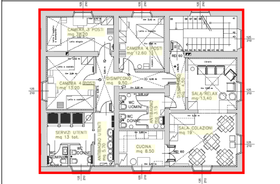
PIANO PRIMO
